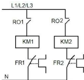
شکل ۱۲. مدار فرمان سیستم بوستر پمپ سه پمپه
